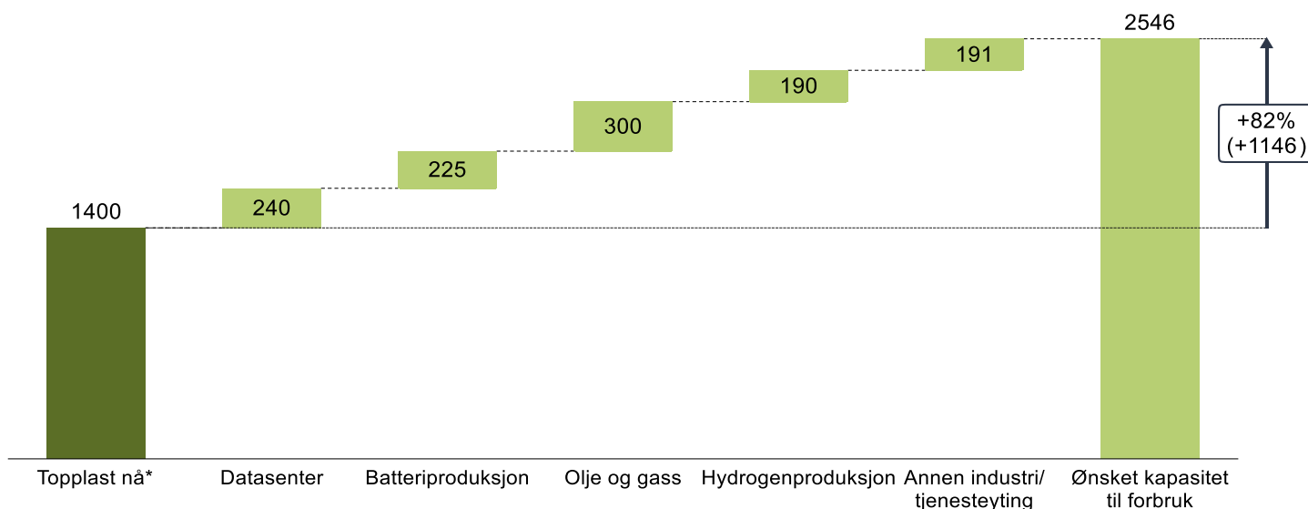
Figur 26 Tilknytningsforespørsler for forbruk hos Lnett i Rogaland, fordelt på forbrukskategori (MW)
