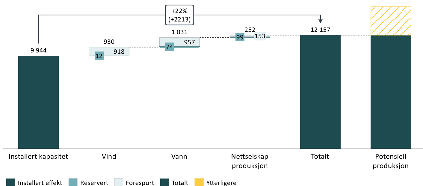
Figur 31 Tilknytningssaker hos Statnett til produksjon (MW).
