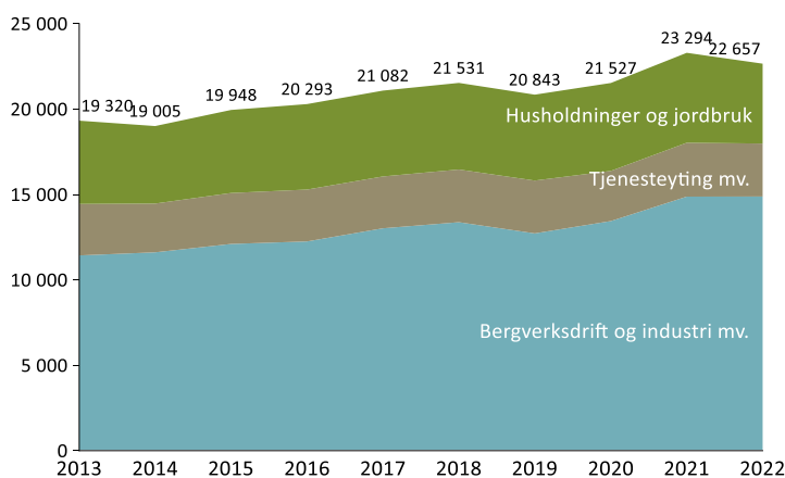
Figur 15 Utvikling i kraftforbruk i Vestland (GWh).
