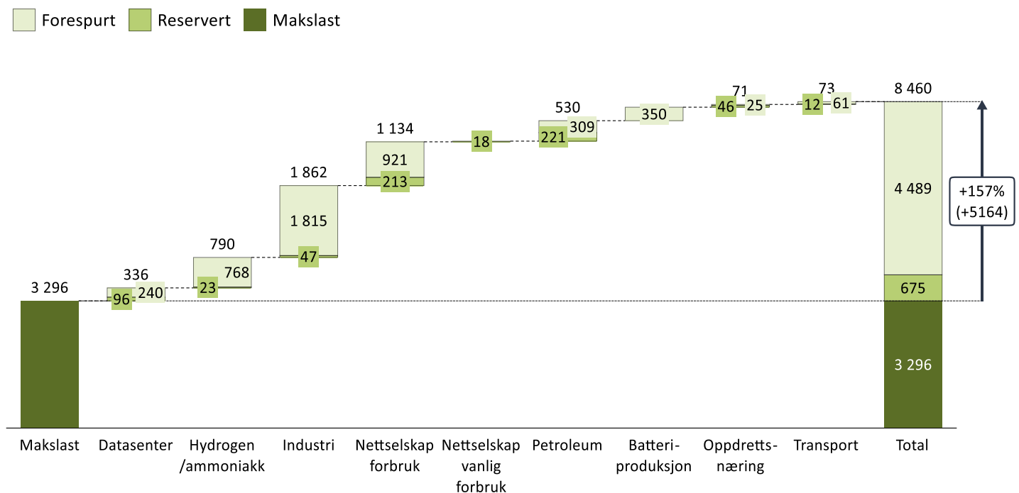
Figur 30 Tilknytningsforespørsler for forbruk hos Statnett i Vestland fordelt på forbrukskategori (MW).
